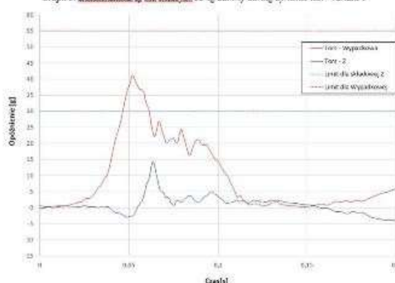
Wykres 7. Przebiegi opóźnienia wypadkowego toru manekina 32 kg podczas testów dynamicznych Graph 7. Decelerations of the chest for 32 kg dummy during dynamic tests
