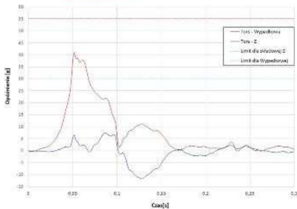
Wykres 4. Przebiegi opóźnień toru manekina 32 kg podczas testu dynamicznego – wariant 1 Graph 4. Decelerations of the chest for 32 kg dummy during dynamic test - variant 1
